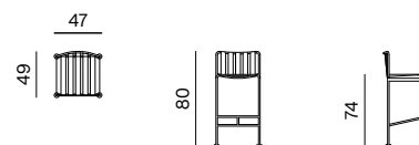
BARSTOOL dimensions 47 x 49 x 80 cm
