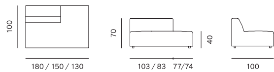
1SEATER EXTENDED (L/R) / 1SJED PRODUŽENI (L/D)
